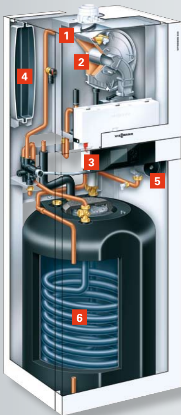
Vitodens 222-F typ FR2B z emaliowanym podgrzewaczem c.w.u. z węzownicą dla obszarów z twardą wodą
